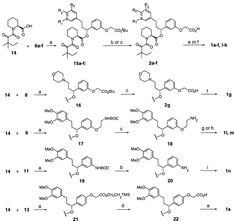
Scheme 2. Reagents and conditions: (a) DCC, DMAP, \text{CH}_2\text{Cl}_2 , 0^\circ\text{C} ; (b) TFA, \text{CH}_2\text{Cl}_2 , 0^\circ\text{C} ; (c) HCl, \text{CH}_2\text{Cl}_2 , 0^\circ\text{C} ; (d) TBAF, DMF, 0^\circ\text{C} ; (e) i. N,N' -disuccinimidyl carbonate, pyridine, \text{CH}_3\text{CN} , 0^\circ\text{C} ; ii. diamine-2HCl, TEA, \text{CH}_3\text{CN} , 0^\circ\text{C} ; (f) diamine, DCC, DMAP, \text{CH}_2\text{Cl}_2 , 0^\circ\text{C} ; (g) CDI, TEA, \text{CH}_2\text{Cl}_2 , 0^\circ\text{C} ; (h) oxalyl chloride, TEA, \text{CH}_2\text{Cl}_2 , 0^\circ\text{C} ; (i) malonic acid, BOP, DIEA, \text{CH}_2\text{Cl}_2 , 0^\circ\text{C} .
